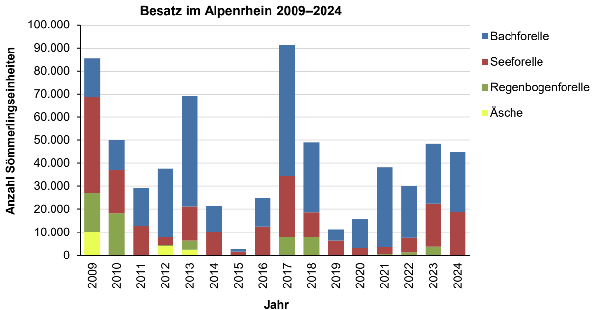
Abb. 13: Standardisierte Angaben zum Besatz im Alpenrhein der Jahre 2009–2024 in Anzahl der Sömmerlingseinheiten.
