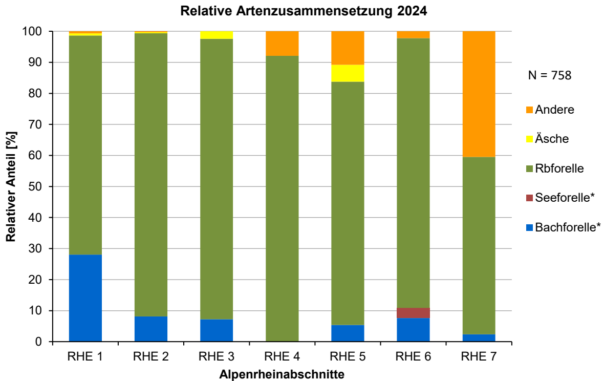
Abb. 4: Relative Artenzusammensetzung des Fangs in den einzelnen Alpenrheinabschnitten 2024. Rbforelle = Regenbogenforelle; *= See- und Bachforellen werden in Graubünden seit 2020 nicht mehr getrennt ausgewiesen.
