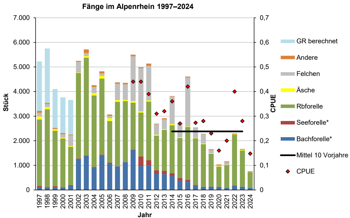
Abb. 10: Gesamtfang im Alpenrhein in den Jahren 1997–2024. Quelle Daten 1997–2007: G. Feuerstein, internationale Strecke. Vor 2002: GR Anteil hochgerechnet von C. Friedl (hellblaue Farbe). Säulen: absolute Fangzahlen; Linie: Zehnjahresmittel der Gesamtfänge der Vorjahre. Ab 2009: Fangzahl pro Fischgang CPUE, catch per unit effort (Skala rechte Achse). *= See- und Bachforellen werden in Graubünden seit 2020 nicht mehr getrennt ausgewiesen).
