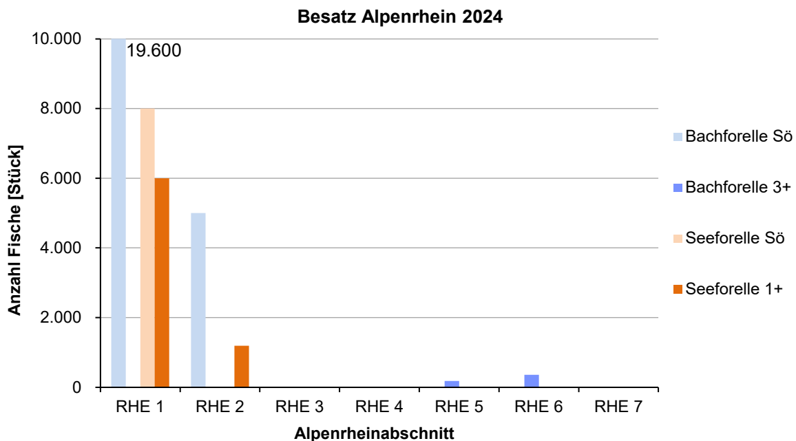
Abb. 11: Fischbesatz (Individuenzahlen), der 2024 direkt in den Alpenrhein erfolgte. Total: 32.330 Stück. Altersklassen: Sö = Sömmerlinge; 1+ = Einjährig; 3+ = 3-jährig.
