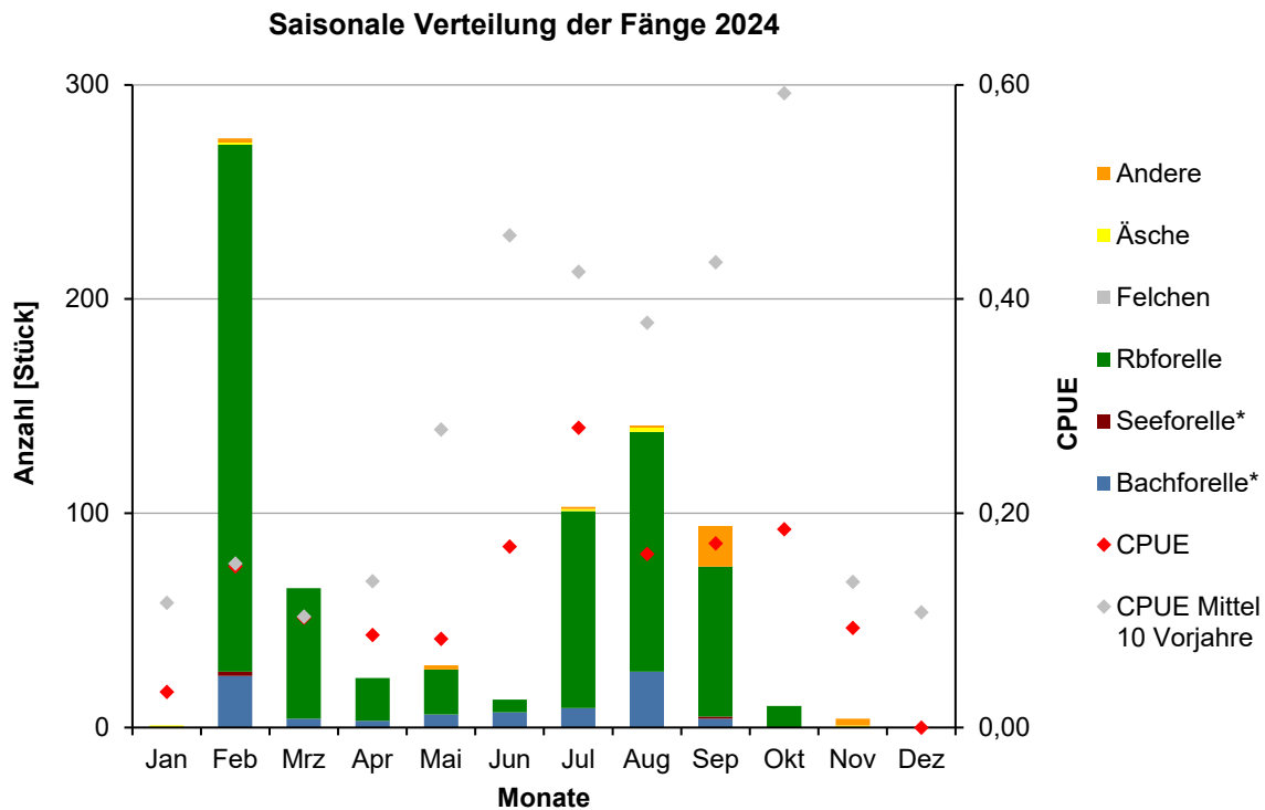
Abb. 7: Saisonale Verteilung der Fänge im gesamten Alpenrhein 2024. CPUE: Rauten auf rechter Skala. Um Vergleiche zu erleichtern, wurden zusätzlich die CPUE-Mittelwerte der zehn Vorjahre dargestellt (graue Rauten). *= See- und Bachforellen werden in Graubünden seit 2020 nicht mehr getrennt ausgewiesen.
