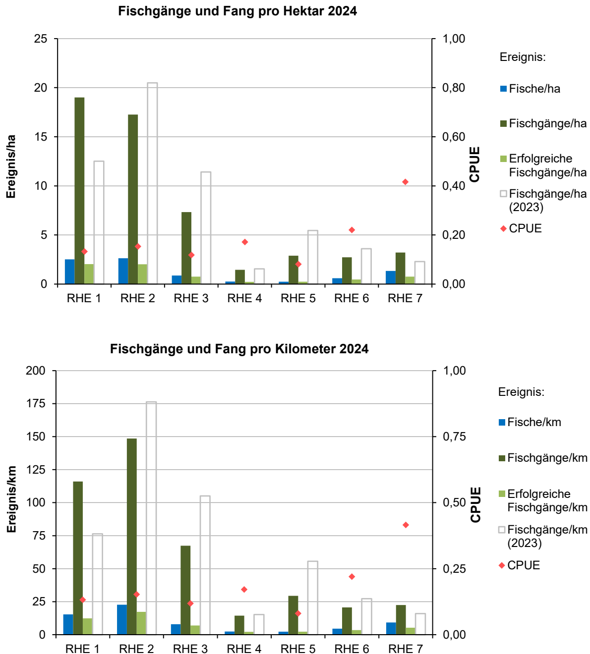
Abb. 6: Anzahl gefangener Fische (Individuen), Anzahl Fischgänge und Anzahl erfolgreicher Fischgänge jeweils pro Hektar (oben) bzw. pro Kilometer Flusslänge (unten) in den sieben Alpenrheinabschnitten sowie der Befischungserfolg in CPUE (catch per unit effort, rechte Skala) 2024. Um Vergleiche zu erleichtern, sind die Daten aus 2023 ebenfalls dargestellt (Fischgänge/ha bzw. Fischgänge/km).
