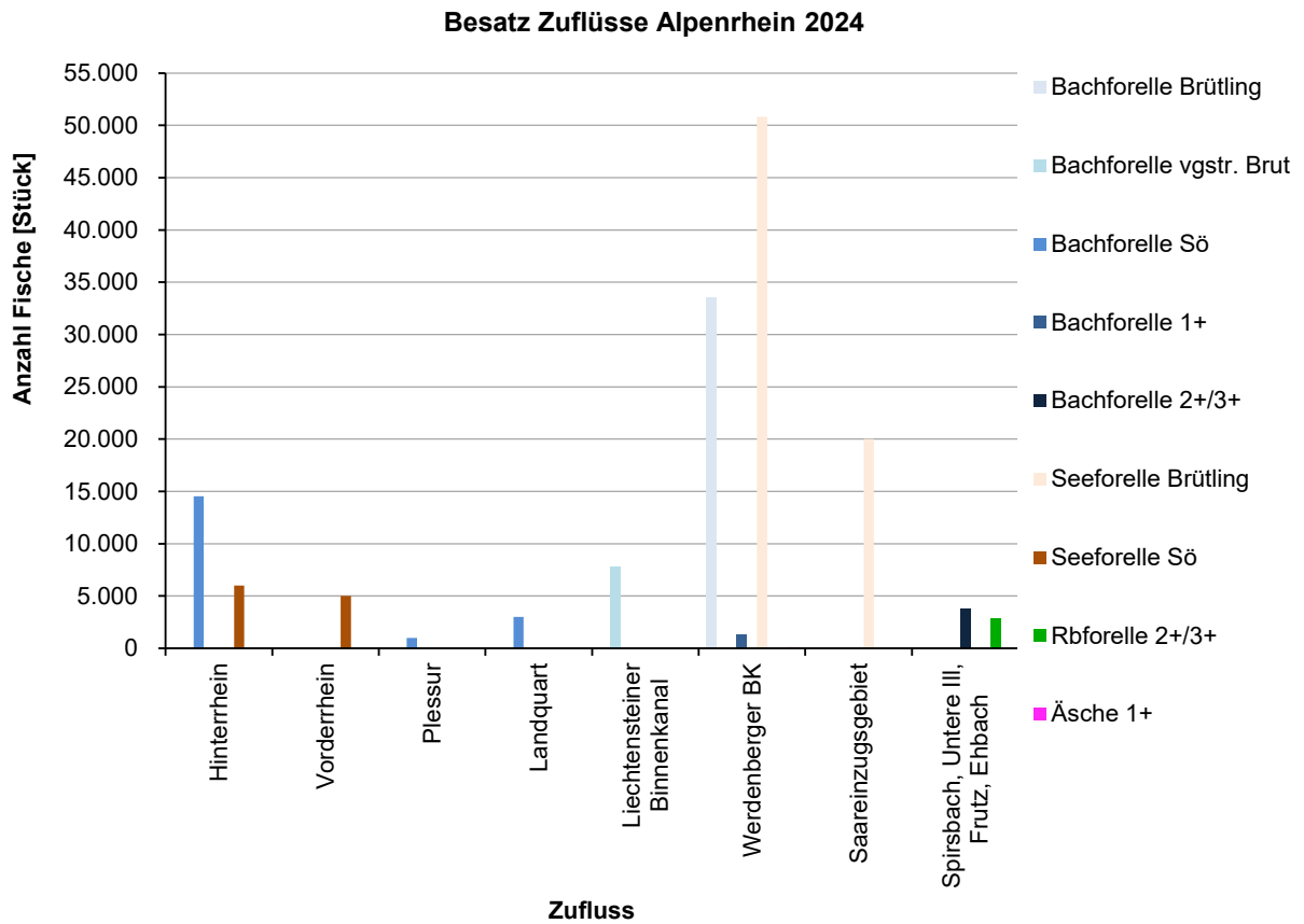
Abb. 14: Fischbesatz (Individuenzahl), der 2024 in die Zuflüsse des Alpenrheins erfolgte. Total: 149.605 Fische. Altersklassen: v.Brut = vorgestreckte Brut; Sö = Sömmerringe; 1+ = 1-jährige; 2+/3+ = 2- bis 3-jährige.
