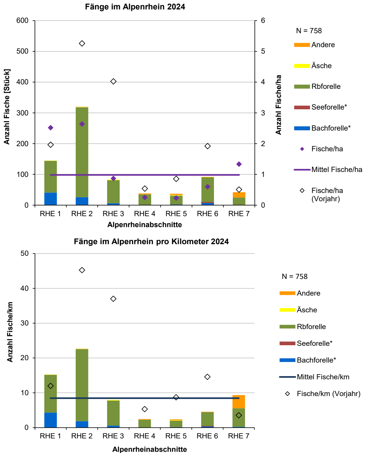
Abb. 3: Fangergebnis in den einzelnen Alpenrheinabschnitten im Jahr 2024 in Individuen, Individuen pro Hektar (rechte Skala in der oberen Abbildung) und Individuen pro Kilometer pro Fischart (untere Abbildung); zu Vergleichszwecken ist in der oberen Abbildung der Ertrag pro Hektar im Vorjahr 2023 und in der unteren Abbildung der Ertrag pro km im Vorjahr (2023) aufgeführt. Rbforelle = Regenbogenforelle; *= See- und Bachforellen werden in Graubünden seit 2020 nicht mehr getrennt ausgewiesen.
