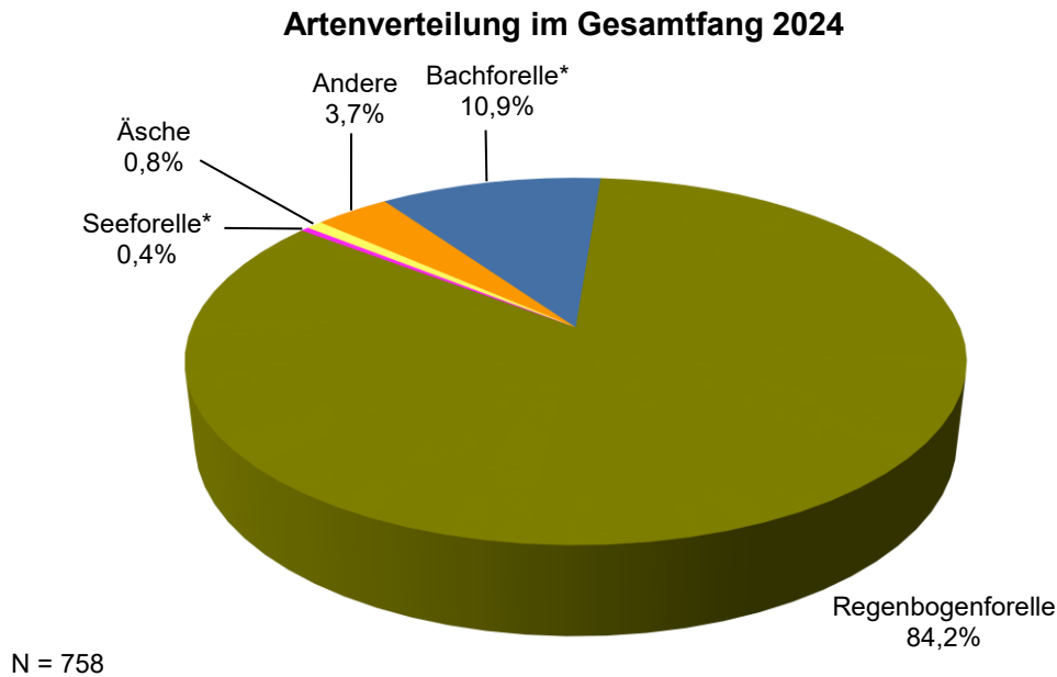
Abb. 2: Artenzusammensetzung des Fangs 2024 im gesamten Alpenrhein. Die Individuenzahl aller gefangenen Fische beträgt 758 (*= See- und Bachforellen werden in Graubünden seit 2020 nicht mehr getrennt ausgewiesen).
