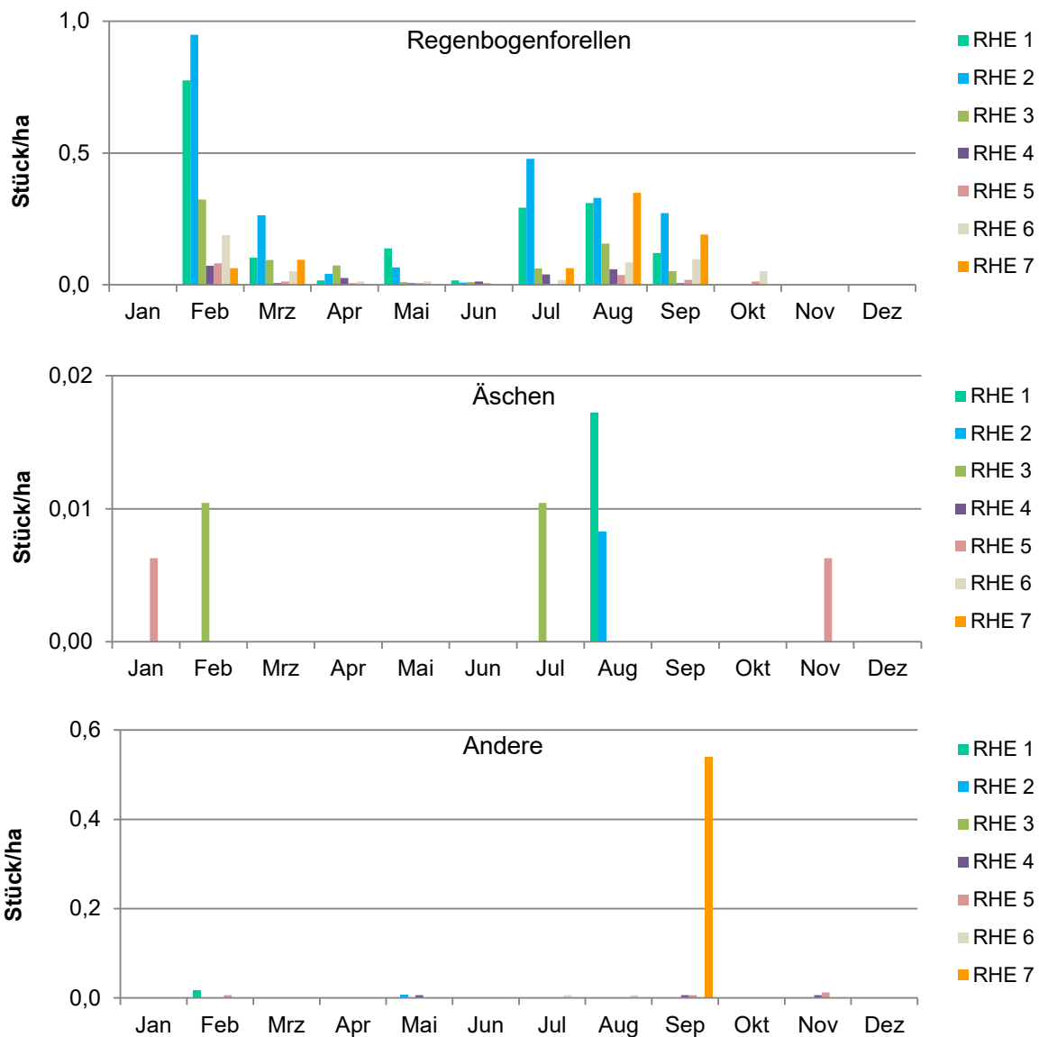
Abb. 9: Saisonale Verteilung der Fänge 2024 nach Fischart in jedem Alpenrheinabschnitt in Individuen pro Hektar (unterschiedliche Y-Achsenkalierung). *= See- und Bachforellen werden in Graubünden seit 2020 nicht mehr getrennt ausgewiesen.
