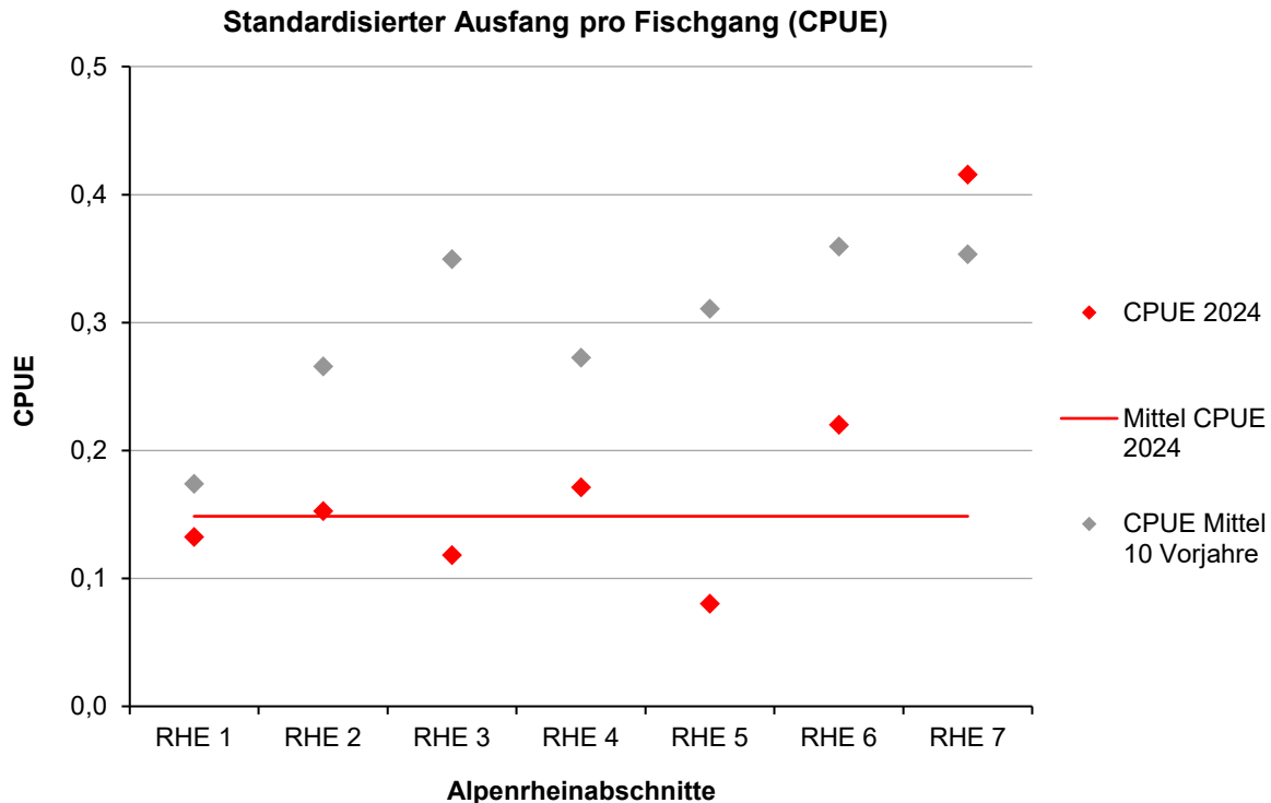
Abb. 5: Fang pro Fischgang (CPUE) in den einzelnen Alpenrheinabschnitten (rote Rauten) sowie der Mittelwert über alle Abschnitte (rote Linie) im Jahr 2024. Um Vergleiche zu erleichtern, wurden zusätzlich die Zehnjahresmittel der CPUE-Werte dargestellt (graue Rauten).
