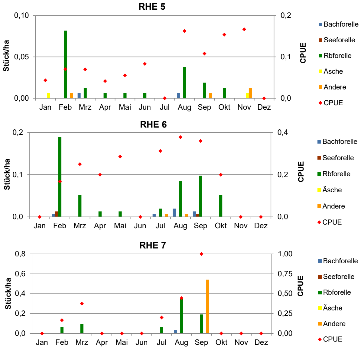
Abb. 8: Verteilung der Fänge im Jahresverlauf in Individuen pro Hektar in den einzelnen Alpenrheinabschnitten (Säulen) im Jahr 2024 (unterschiedliche Y-Achsenkalierung). Fang pro Fischgang, CPUE (Punkte, rechte y-Achse). *= See- und Bachforellen werden in Graubünden seit 2020 nicht mehr getrennt ausgewiesen.
