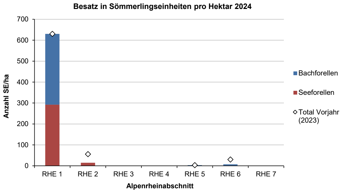
Abb. 12: Standardisierte Angaben zum Besatz in den Alpenrhein in Sömmerlingseinheiten pro Hektar für das Jahr 2024 nach Arten (Säulen) und als Total der Sömmerlingseinheiten aller Arten pro Hektar für das vorherige Jahr 2023 (Rauten). Rbforelle = Regenbogenforelle.
