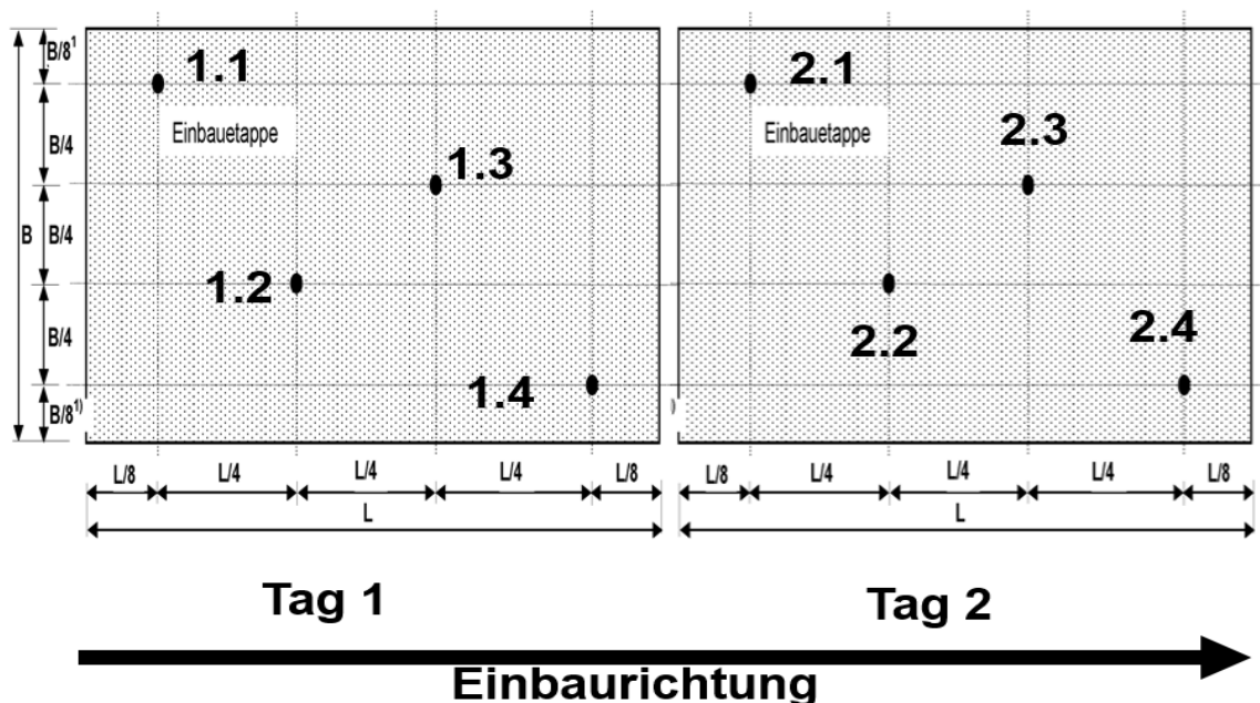
Abbildung: Entnahmeplan für Bohrkern
