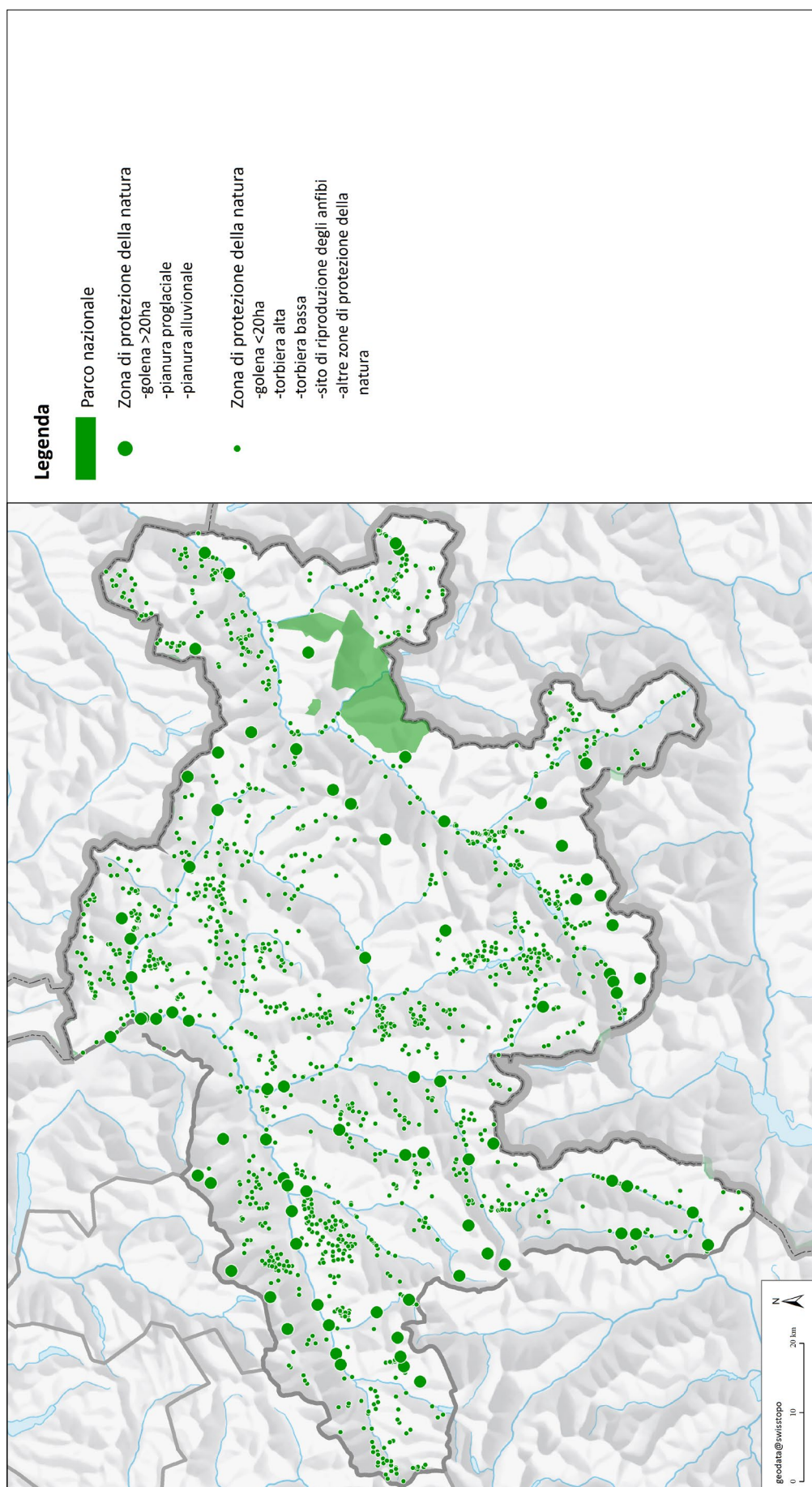
Illustrazione 3.13: Panoramica delle zone di prote- zione della natura
